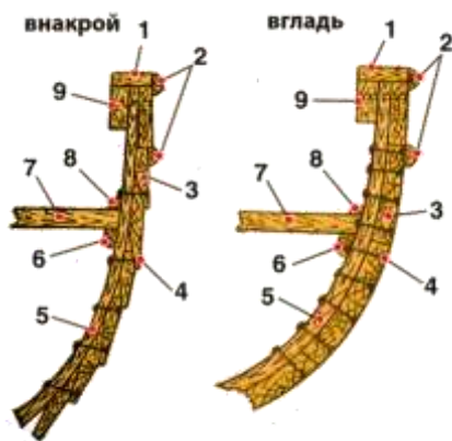
Рис. 8 Обшивка
