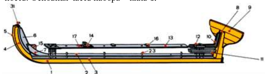
Рис. 3 остов шлюпки
