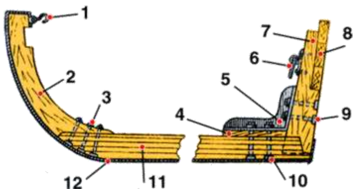
Рис. 4 остов шлюпки.
