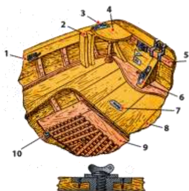
Рис 9 устройство кормы.
