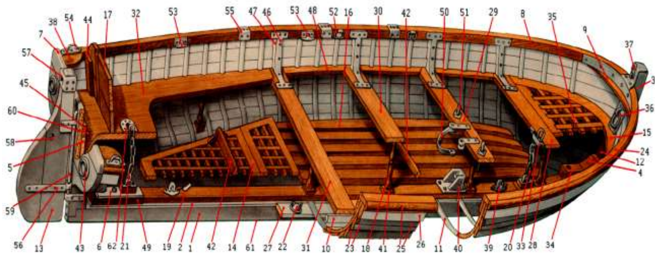
Рис. 2 устройство шестивесельного яла.
