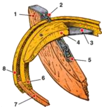
Рис. 7 крепление привального бруса
