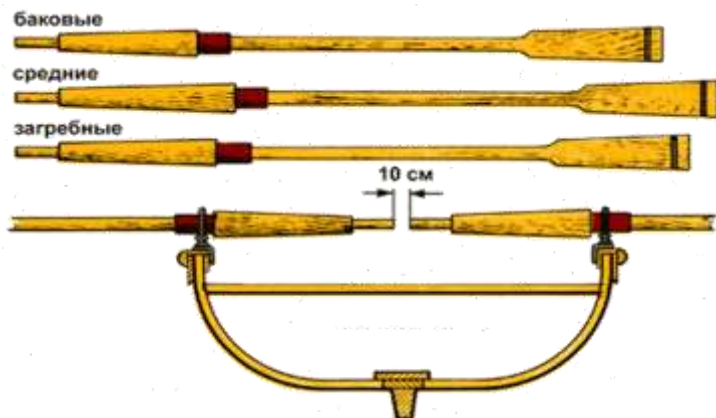
Рис. 16 Положение весел
