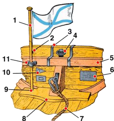
Рис. 10 корма.
