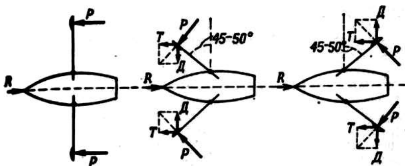
Рис. 23. Силы, действующие на шлюпку при гребле
