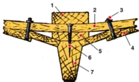
Рис. 6 крепление шпангоутов
