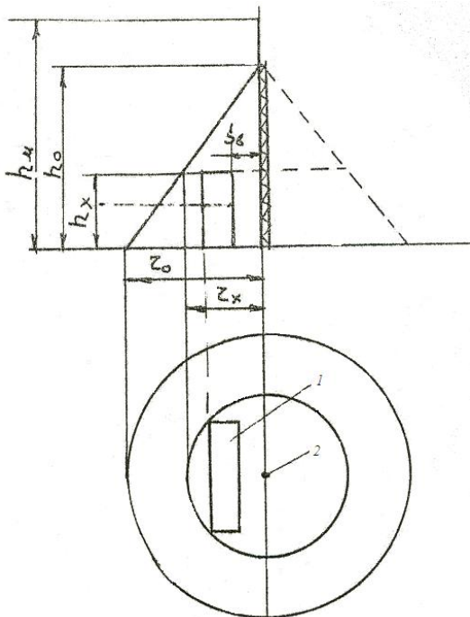
Рис. 1. Молниеотвод:
