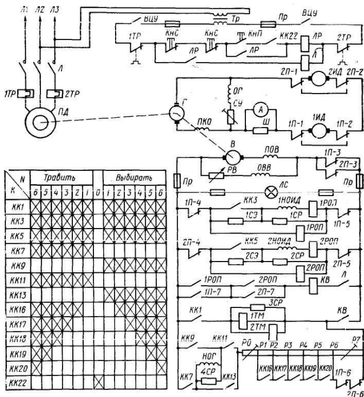
Рис. 3.246. Схема электропривода брашпиля по системе Г – Д
