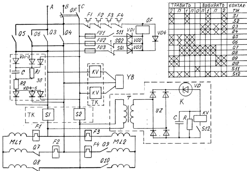
Рис. 3.244. Схема контроллера с бестоковой коммутацией для управления двухскоростным ЭД
