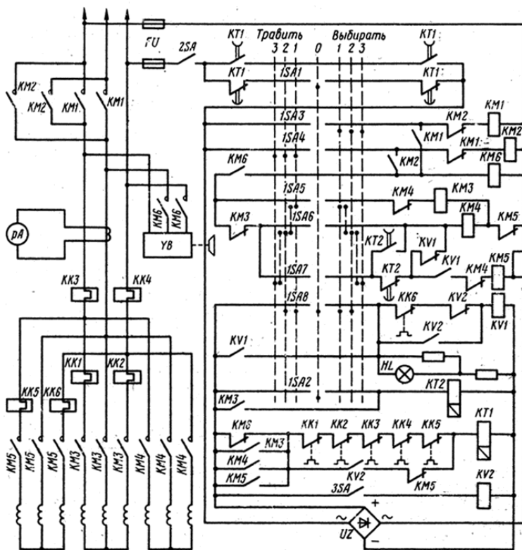
Рис. 3.243. Схема типовой контроллерной системы управления электроприводом якорно-швартовного устройства на переменном токе
