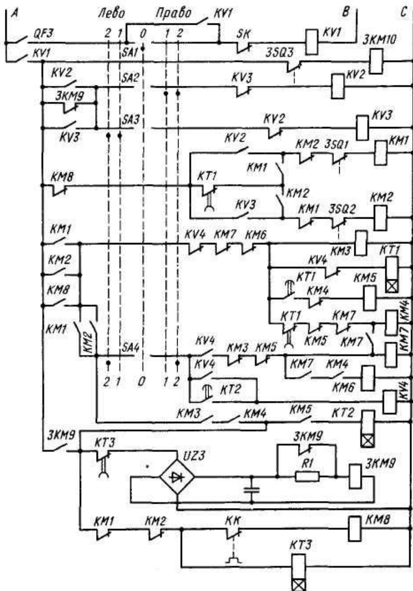
Рис. 3.250. Схема управления механизмом поворота крана
