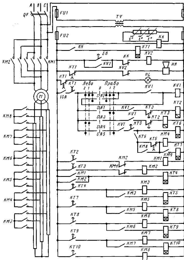
Рис. 3.252 Принципиальная схема электропривода подруливающего устройства
