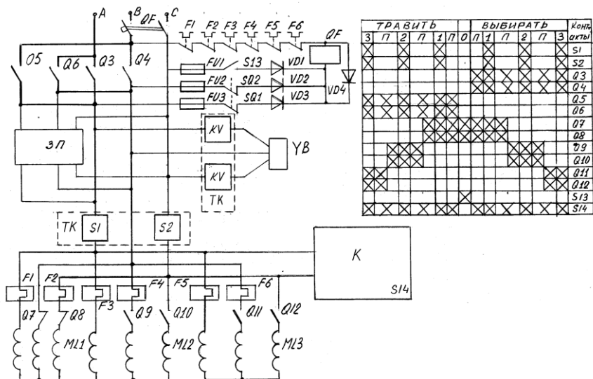
Рис. 3.245. Схема контроллера с бестоковой коммутацией для управления трехскоростным ЭД
