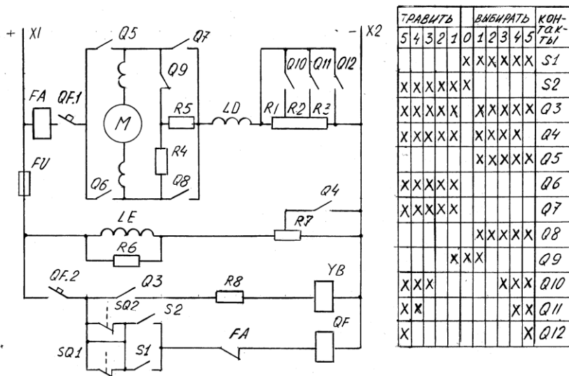
Рис. 3.239. Схема электропривода с кулачковым контроллером KB1200
