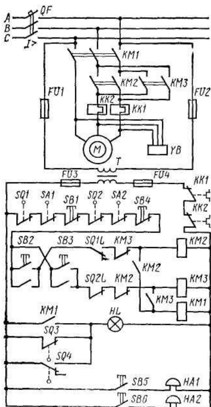
Рис. 3.247. Принципиальная схема электропривода односкоростного лифта на 2 остановки
