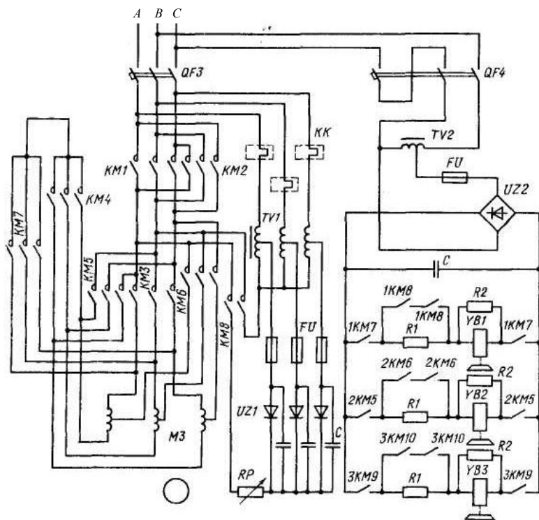
Рис. 3.249. Схема включения катушек электромагнитных тормозов крана
