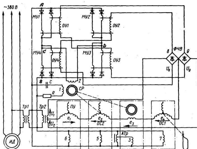
Рис. 3.238. Схема следящего управления РЭП судов типа «А. Пушкин»
