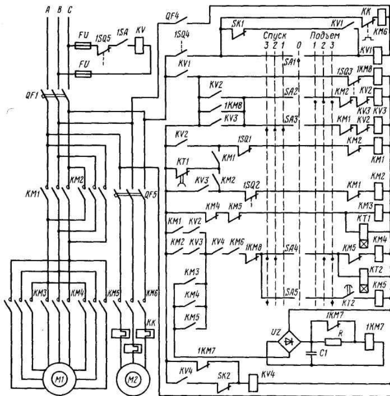
Рис. 3.248. Схема управления механизмом подъема груза грузового крана
