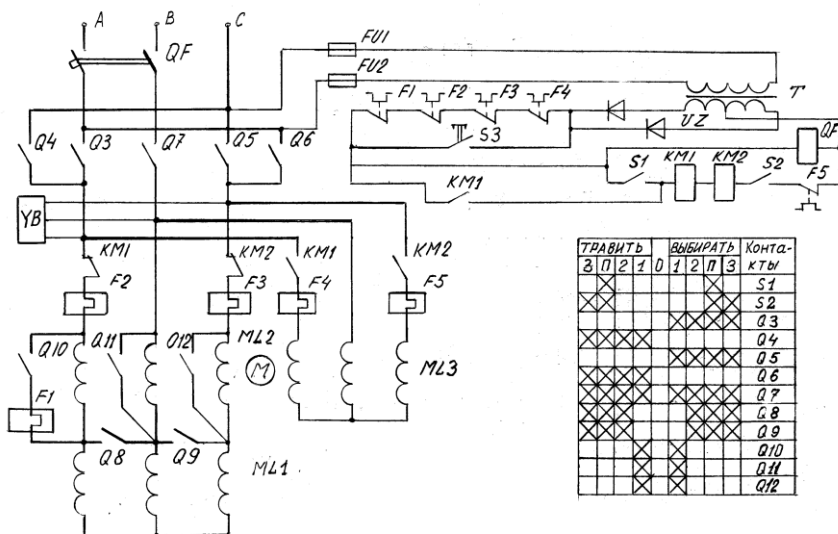
Рис. 3.242. Схема электропривода с кулачковыми контролером KB-2000
