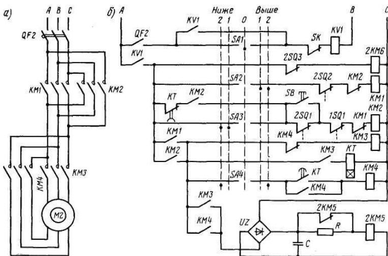
Рис. 3.251. Схема управления механизмом изменения вылета стрелы крана
