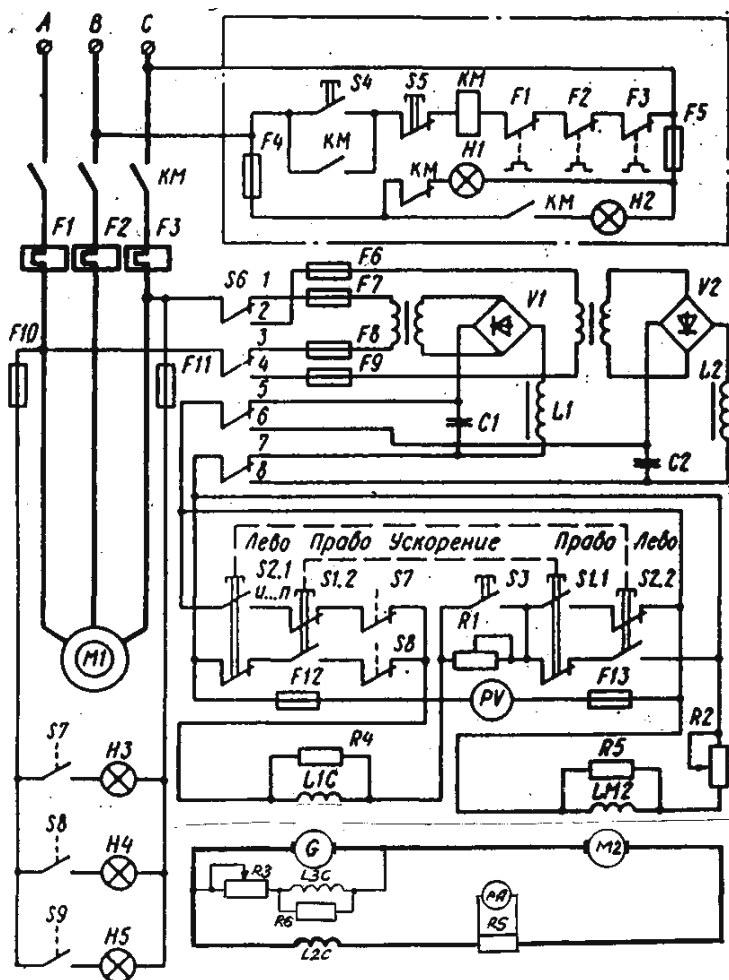
Рис. 3.237. Схема простого управления РЭП судов типа «Волго-Балт»
