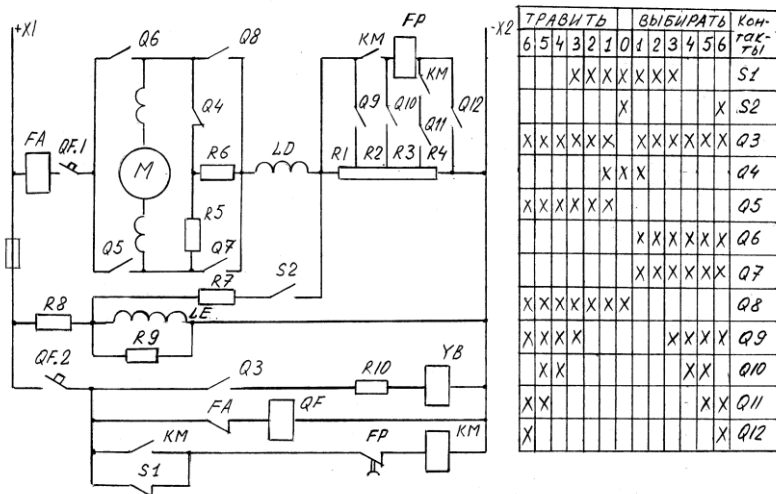
Рис. 3.240. Схема электропривода с кулачковым контроллером KB2500
