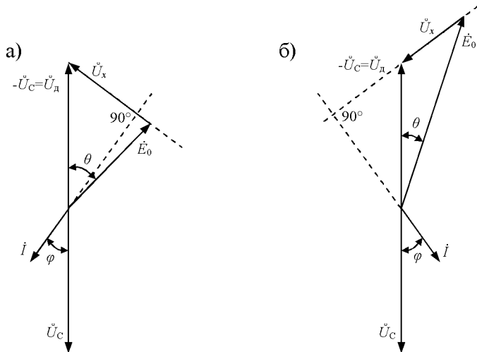
Рис. 4.6. Векторная диаграмма электрических параметров синхронного двигателя: а – недовозбуждение; б – перевозбуждение
