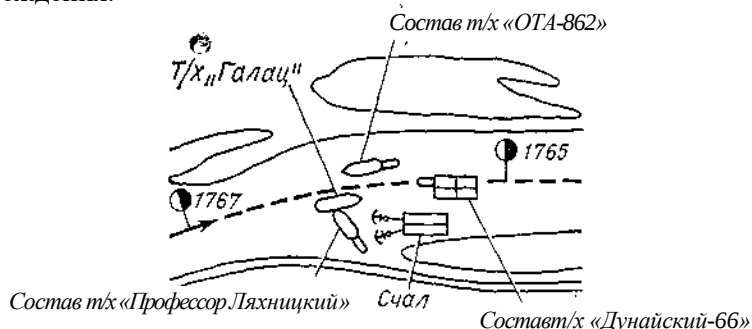
Схема столкновения теплохода «Галац» с составом теплохода «Профессор Ляхницкий»
