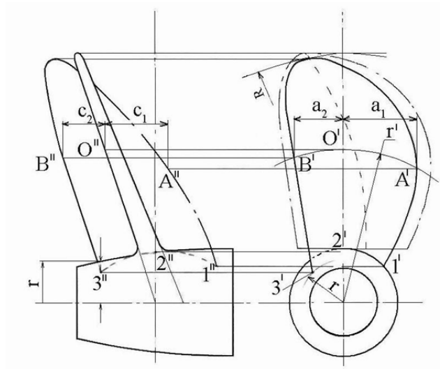
Рис. 4.5. Построение проекций лопасти
