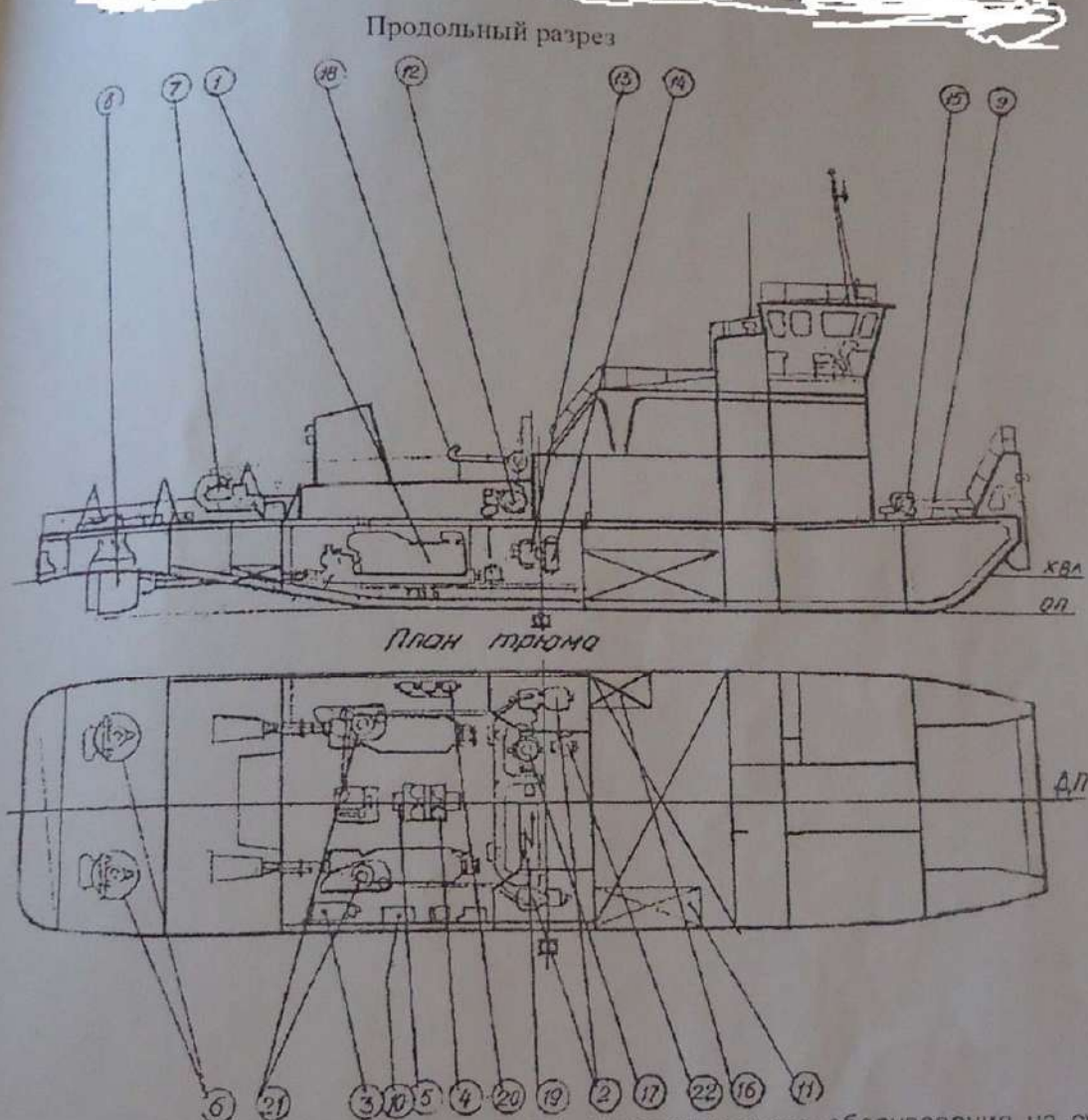
Рис. Схема расположения основного энергетического оборудования на судне. 1 - гл. двигатель; 2 - дизель-генератор; 3 - котлоагрегат; 4 - баллоны сжатого воздуха; 5 - компрессор; 6 - рулевые машины; 7 - буксирная лебедка; 8 - движительно-рулевой комплекс; 9 - автосцеп; 10 - расходный бак; 11 - бак основного запаса топлива; 12 - вентилятор; 13 - теплообменник; 14 - гидрофор; 15 - брашпиль; 16 - сточно-фановая цистерна; 17 - пожар. насос; 18 - сан. насос; 19 - ГРЩ; 20 - маслопрокачив. насосы; 21 - утилизационные котлы; 22 - осушительный насос.
