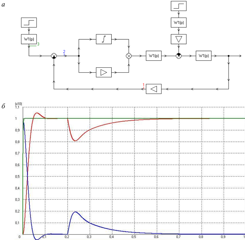
Рис. 2.2. Схема модели ( a ) и результаты моделирования ( б )
