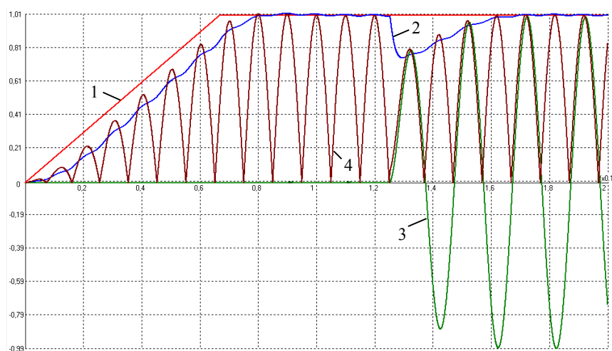
Рис. 3.8. Переходный процесс в генераторе при набросе нагрузки с \cos\varphi=1
