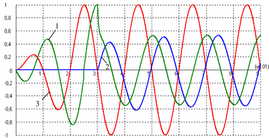
Рис. 3.4. Переходный процесс в генераторе при \cos\varphi=0,3
