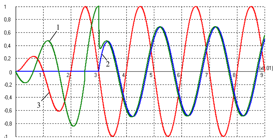
Рис. 3.2. Переходный процесс в генераторе при \cos\varphi=1
