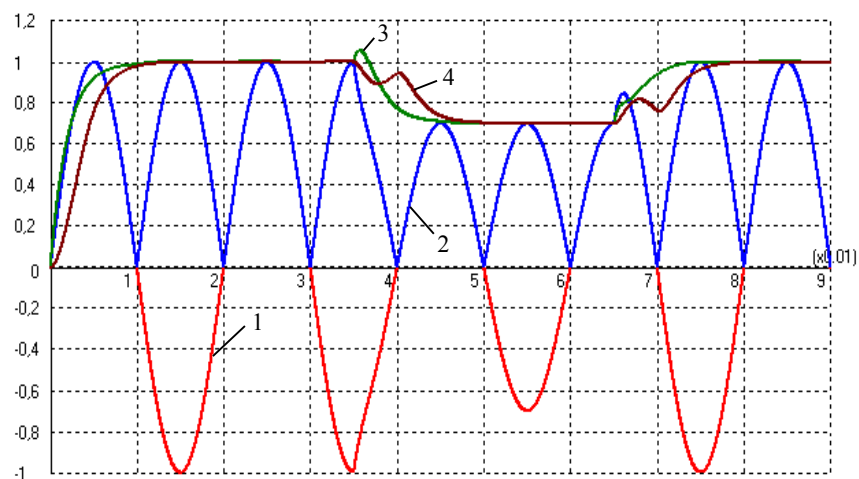
Рис. 3.6. Переходный процесс в преобразователе на базе дифференцирующего устройства и устройства сдвига для t=0,035 с
