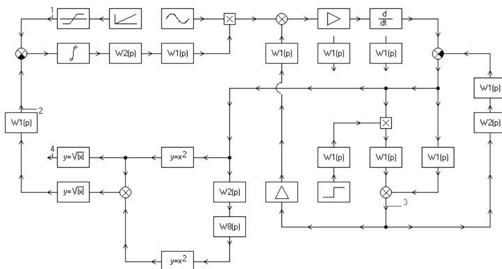
Рис. 3.7. Структурная схема моделей замкнутой системы регулирования напряжения генератора
