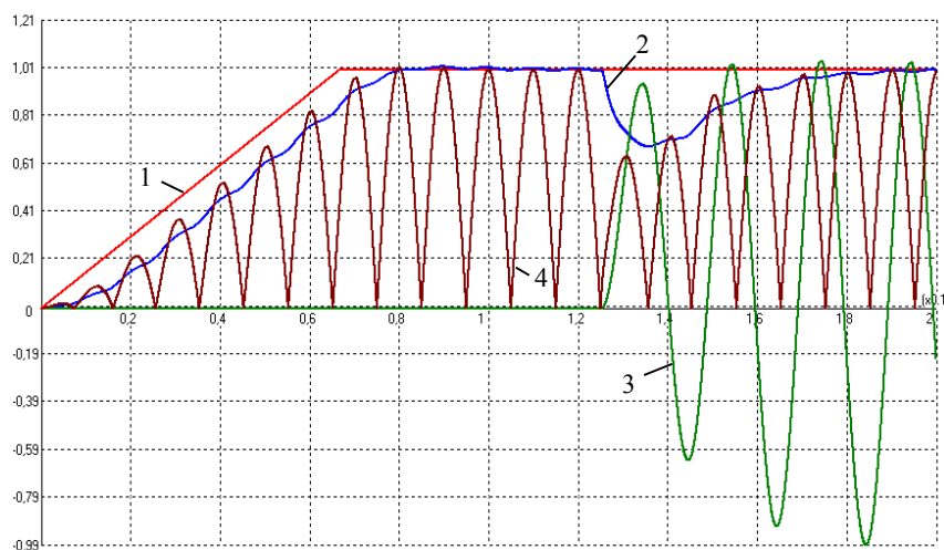
Рис. 3.10. Переходный процесс в генераторе при набросе нагрузки с \cos \varphi = 0.3
