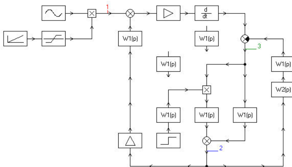
Рис. 3.1. Структурная схема модели неявнополюсного синхронного генератора
