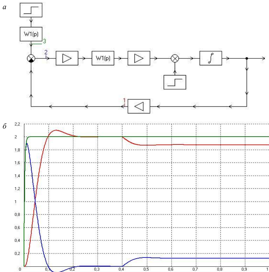
Рис. 2.3. Схема модели ( a ) и результаты моделирования ( б )
