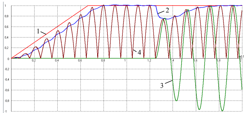
Рис. 3.9. Переходный процесс в генераторе при набросе нагрузки с \cos \varphi = 0.8
