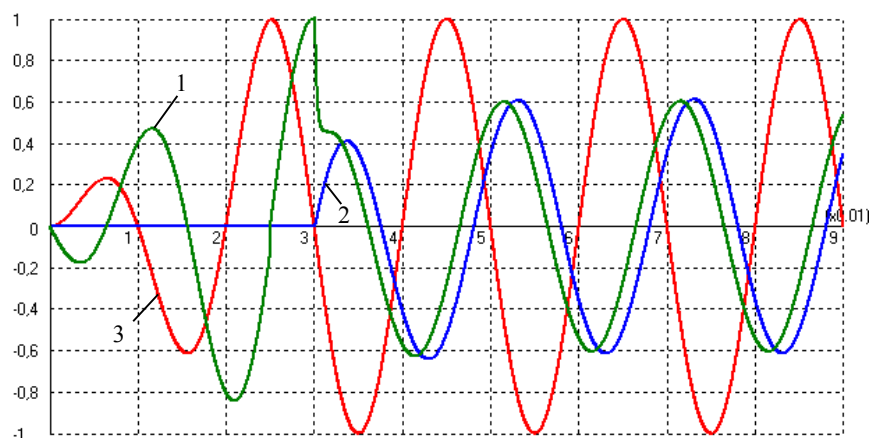
Рис. 3.3. Переходный процесс в генераторе при \cos\varphi=0,8
