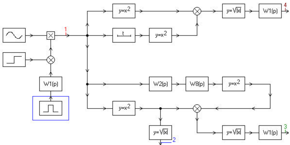
Рис. 3.5. Структурная схема модели устройств преобразования напряжения генератора
