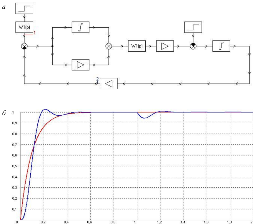
Рис. 2.4. Схема модели ( a ) и результаты моделирования ( б )
