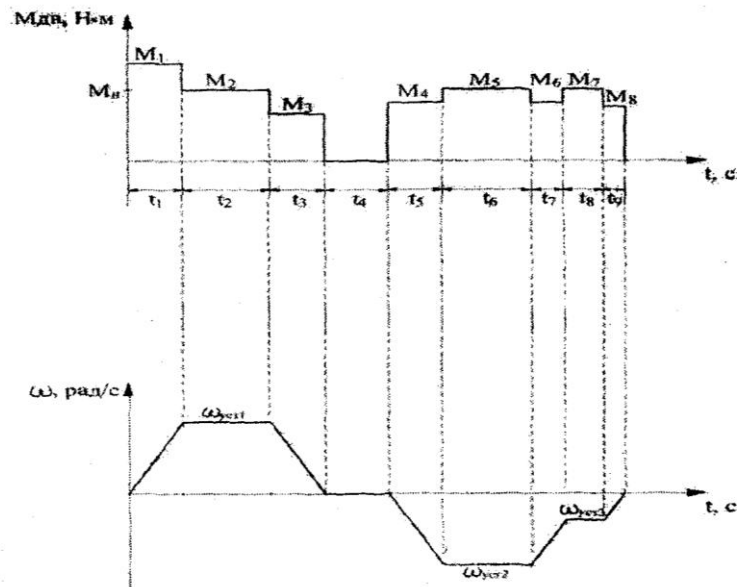
Рис. 4. Нагрузочная диаграмма и тахограмма грузоподъёмного механизма
