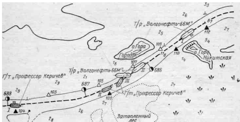
Схема столкновения грузового теплохода «Профессор Керичев» с танкером «Волгонефть-66М»
