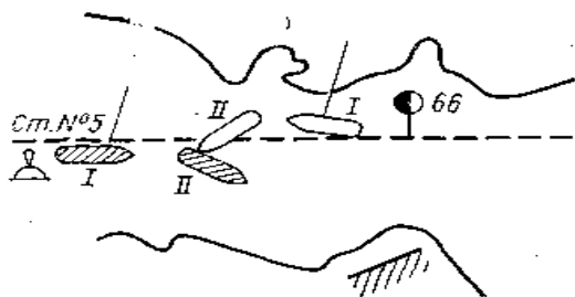
Схема столкновения теплохода «Кизляр» с теплоходом «Кашира»
