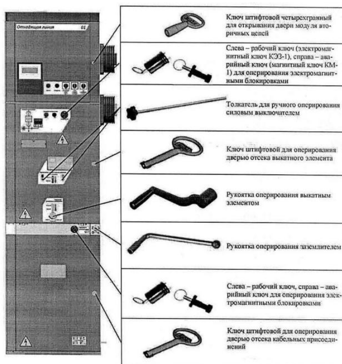
Рис. 1 Принадлежности КРУ
