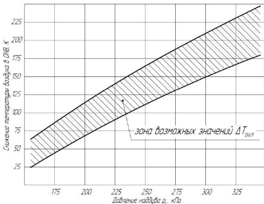
Рис. 1. График для выбора значения \Delta T_{\text{охл}}
