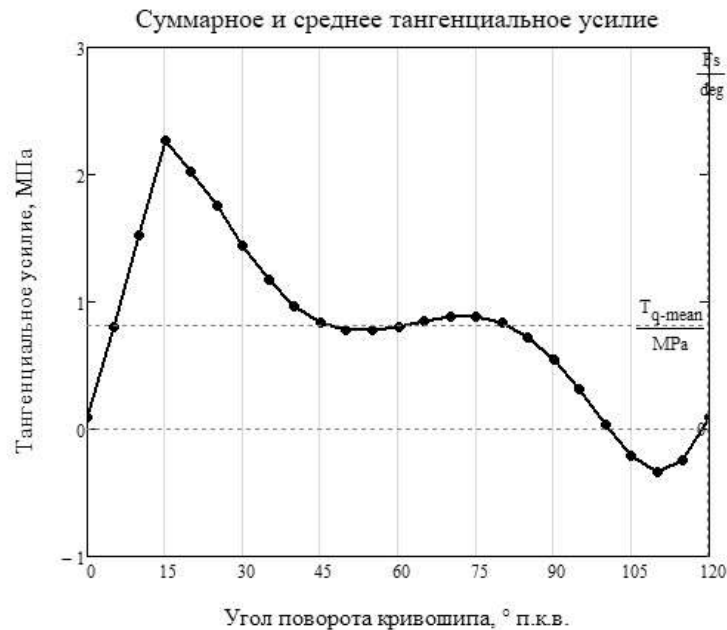
Рисунок – Определение среднего тангенциального усилия
