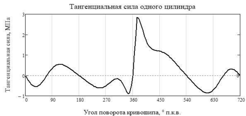
Рисунок – Тангенциальная сила одного цилиндра
