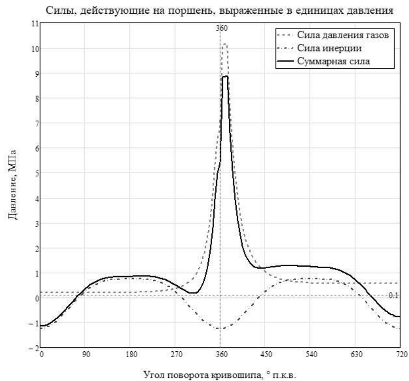
Рисунок – Силы, действующие на поршень
