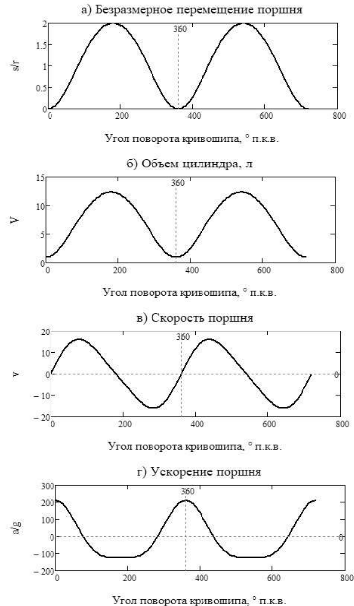
Рисунок – Кинематические параметры двигателя
