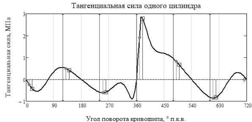
Рисунок – Способ определения суммарного тангенциального усилия (сначала суммируются все ординаты, показанные закрасненными кружками, затем незакрасненными квадратами и т.д.)
