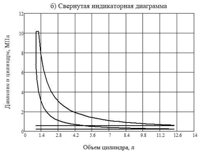
Рисунок – Индикаторные диаграммы
