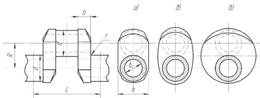
Рисунок 1 – Колена вала с различной формой щек: а – призматическая; б – овальная; в – цилиндрическая.
