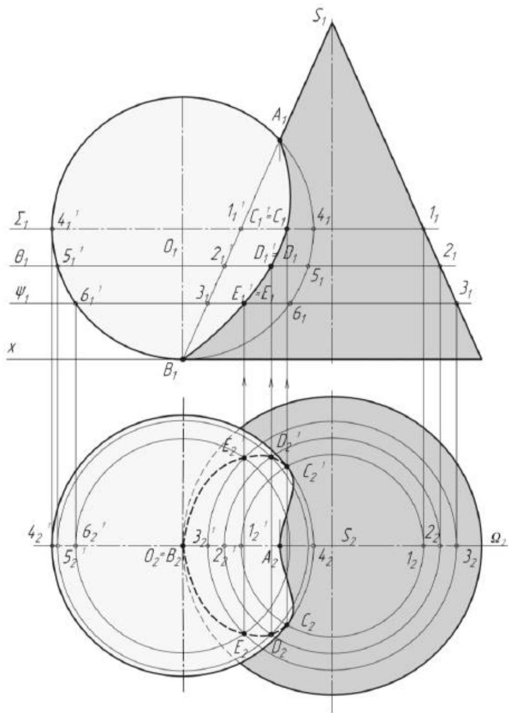
Рис.3. Построение линии пересечения тел секущими плоскостями уровня
