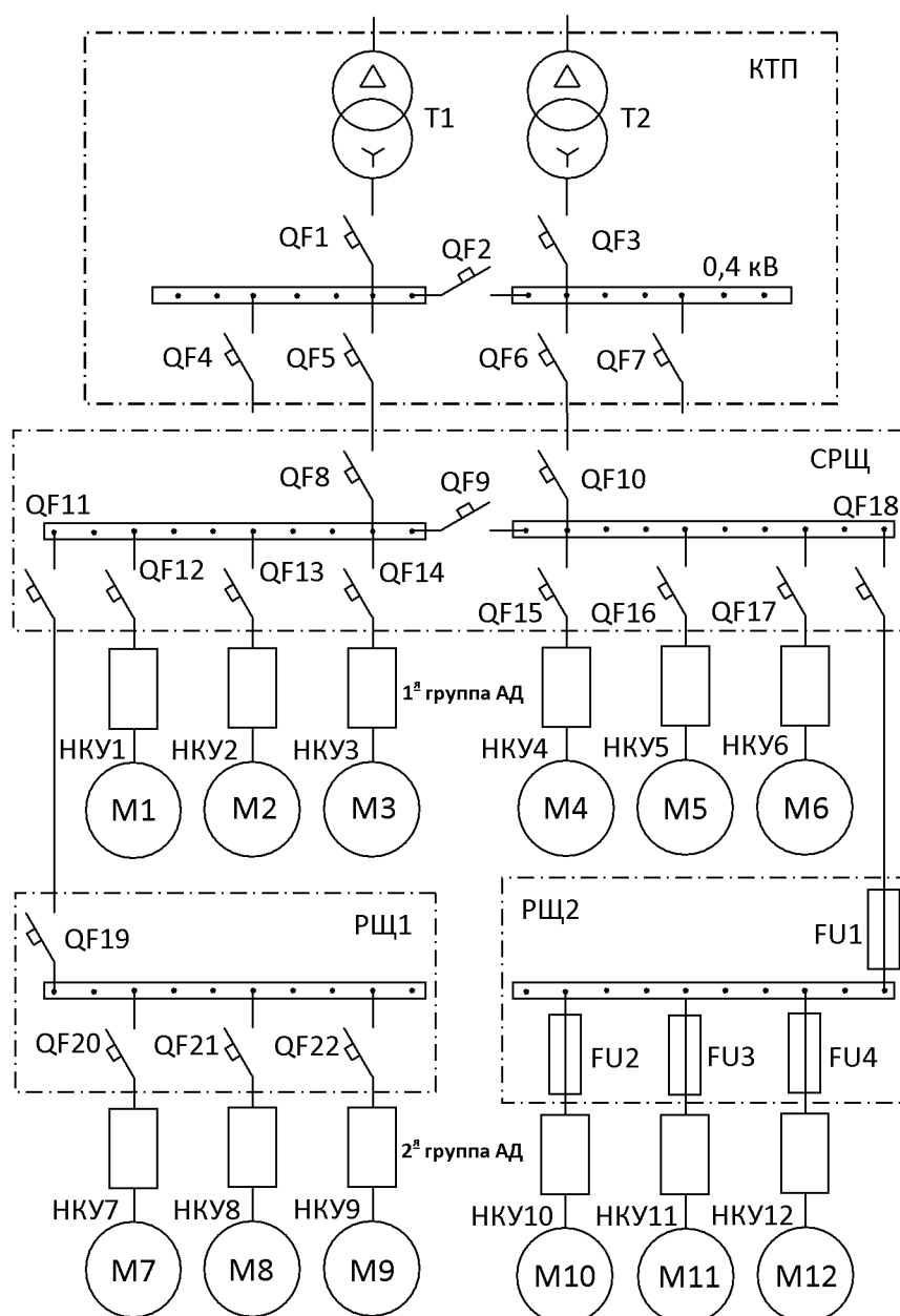
Рис. 1.1. Радиальная трехступенчатая схема электроснабжения
