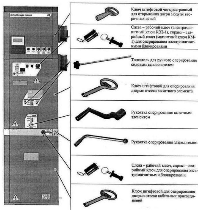
Рис. 1 Принадлежности КРУ
