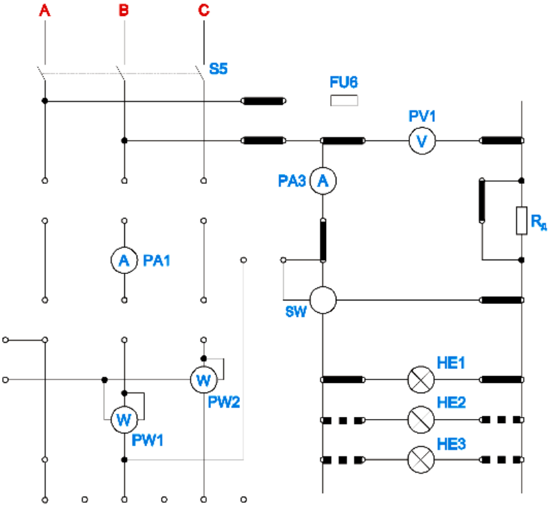
Рисунок 4.1а Монтажная схема для следования однофазного счетчика для нагрузок до 25%
