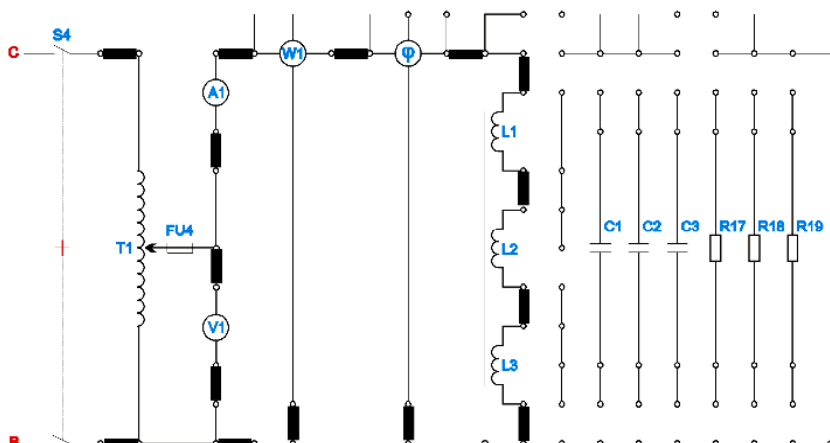
Рисунок 3.2 Монтажная схема для исследования ваттметра по углу рассогласования
