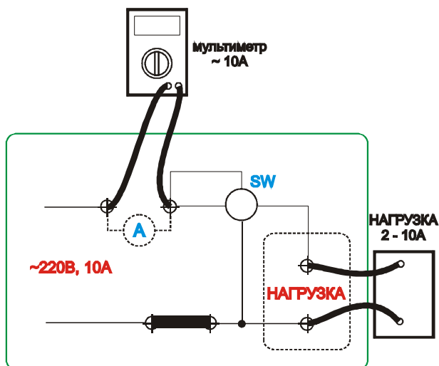
Рисунок 4.1б Монтажная схема для следования однофазного счетчика для нагрузок более 25%
